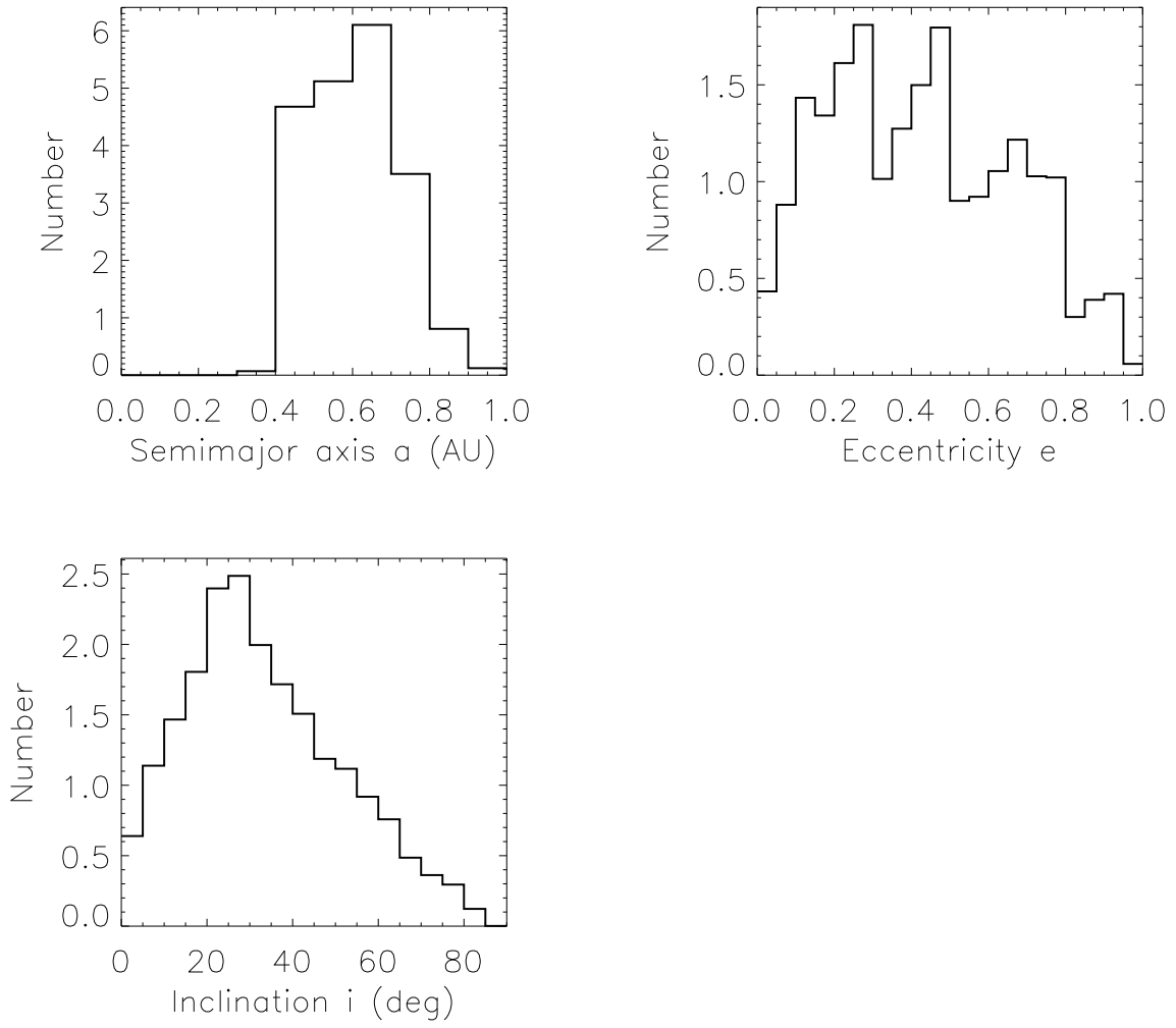
Fig. 16.— IEOs.
