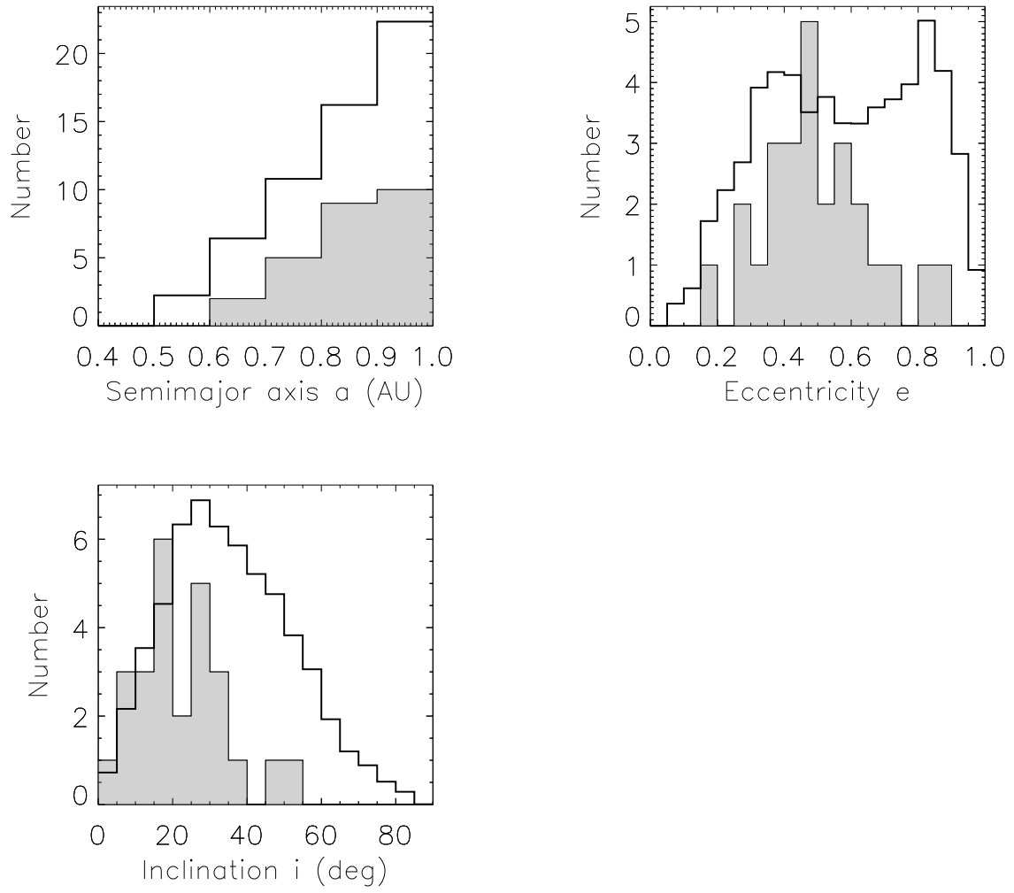
Fig. 15.— Atens.
