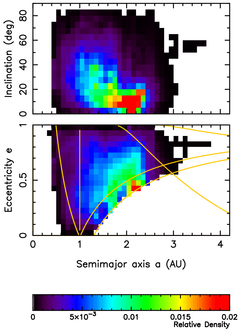
Fig. 3.— \nu_6 resonance
