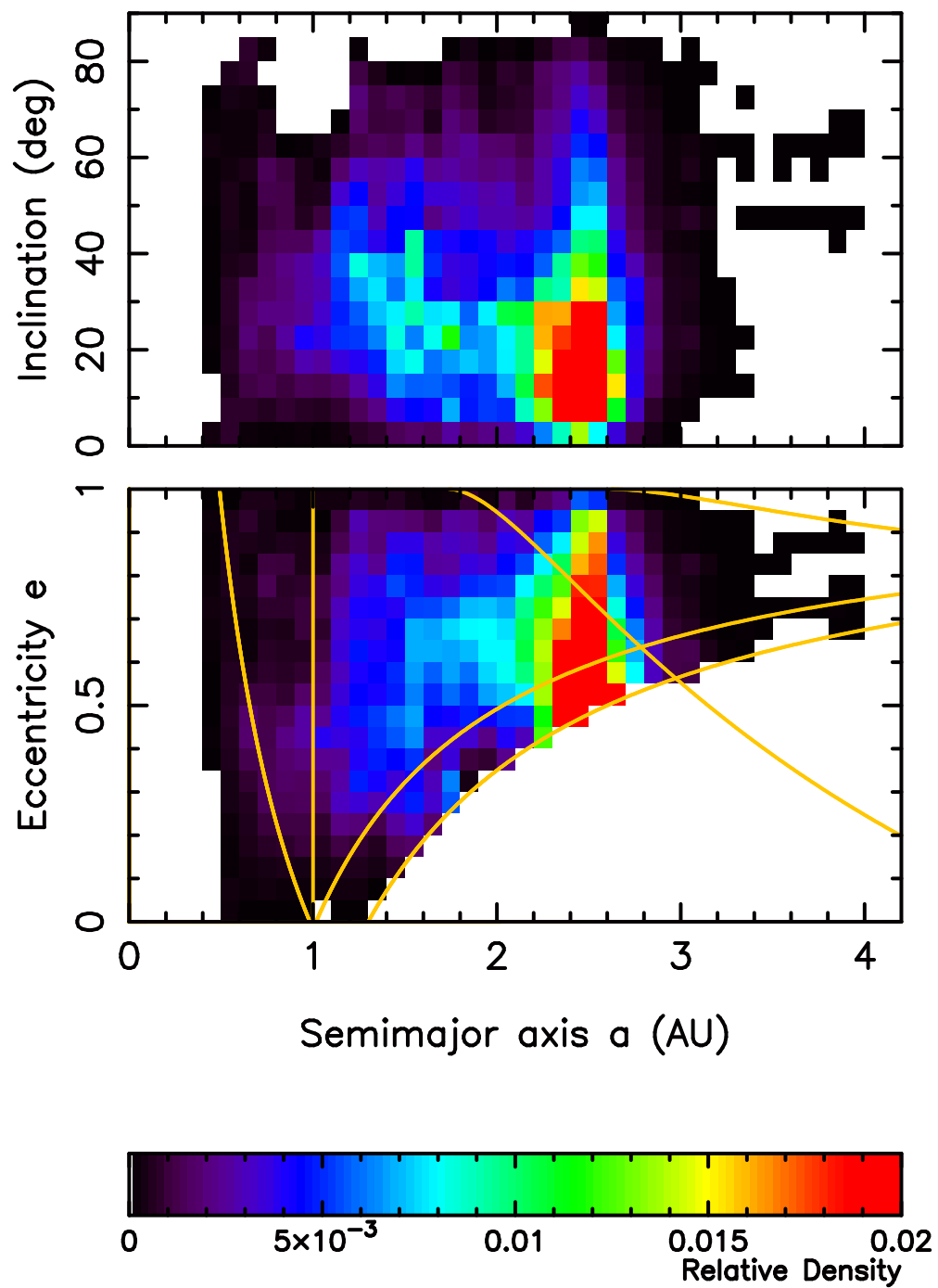
Fig. 2.— 3:1 resonance
