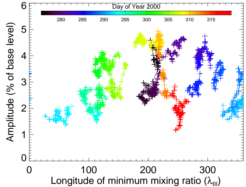
O II Dawn Ansa
