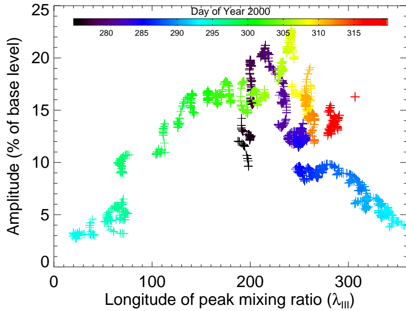
S IV Dawn Ansa
